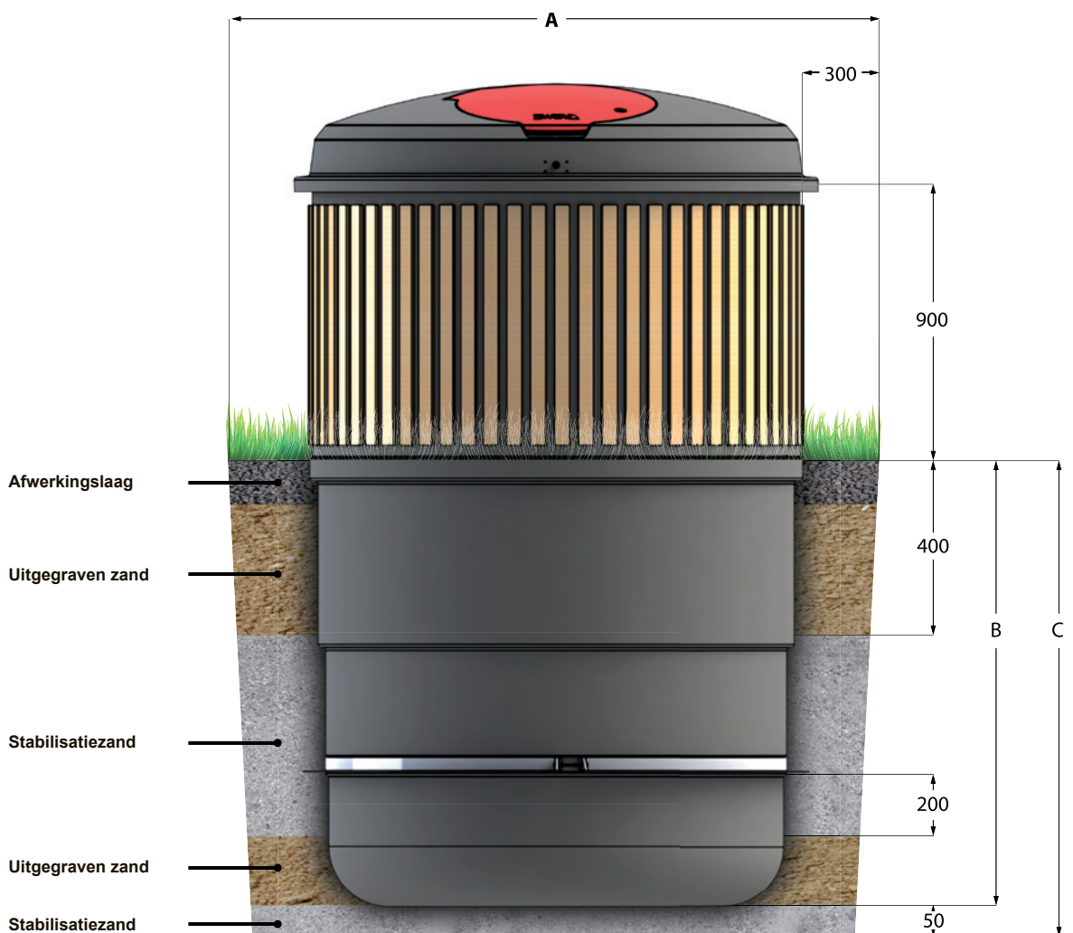
figuur 1. Z-Bin container met de verschillende lagen zand voor de installatie
