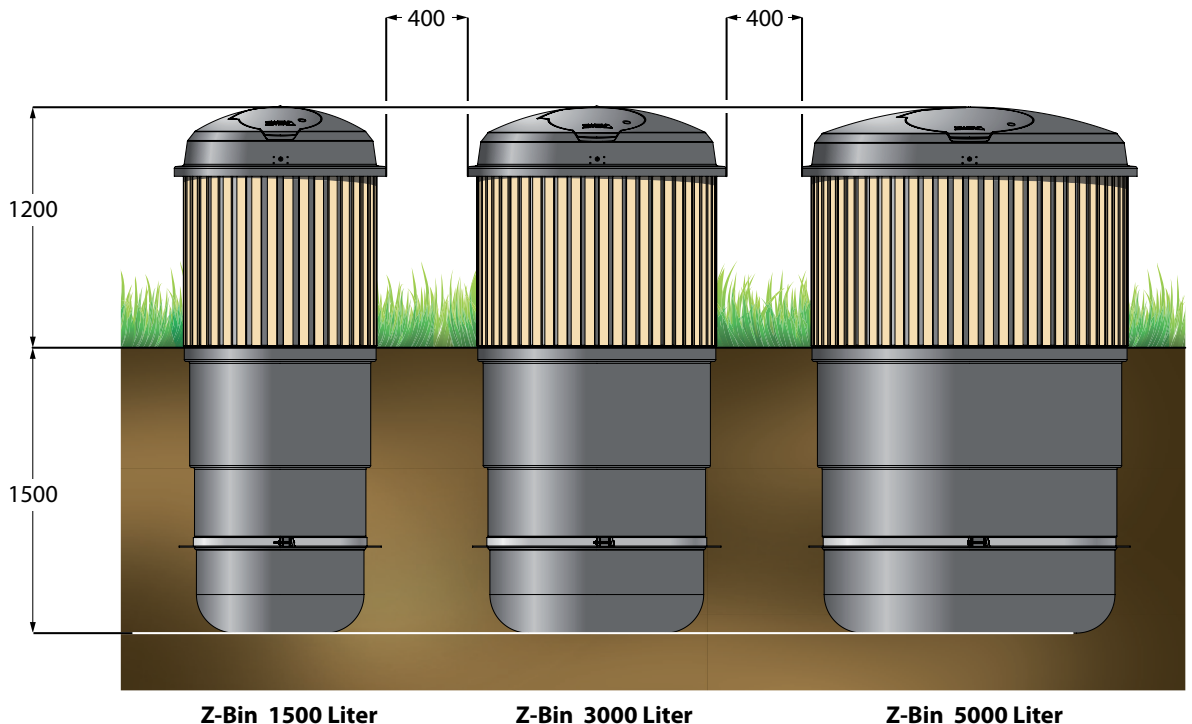
figuur 2. Z-Bin container familie met de onderlinge afstanden en diepte en hoogte
