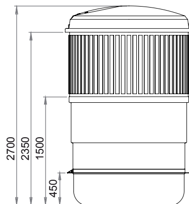
zijaanzicht
