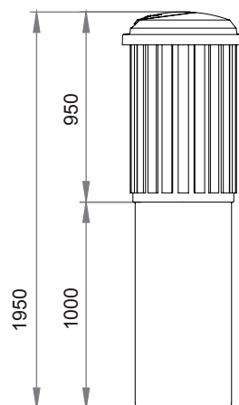
zijaanzicht
