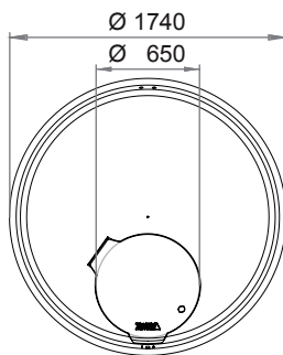
Bovenaanzicht
