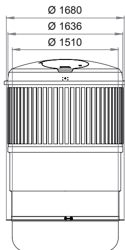
vooraanzicht
