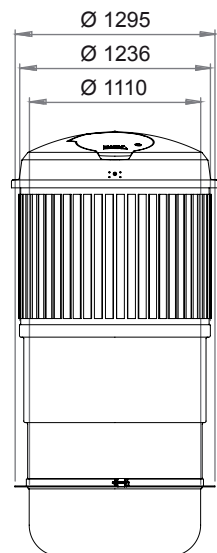
vooraanzicht
