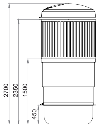
zijaanzicht
