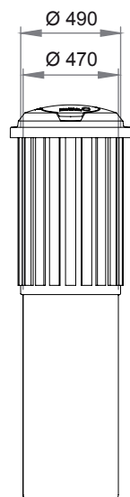
vooraanzicht
