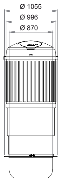
vooraanzicht
